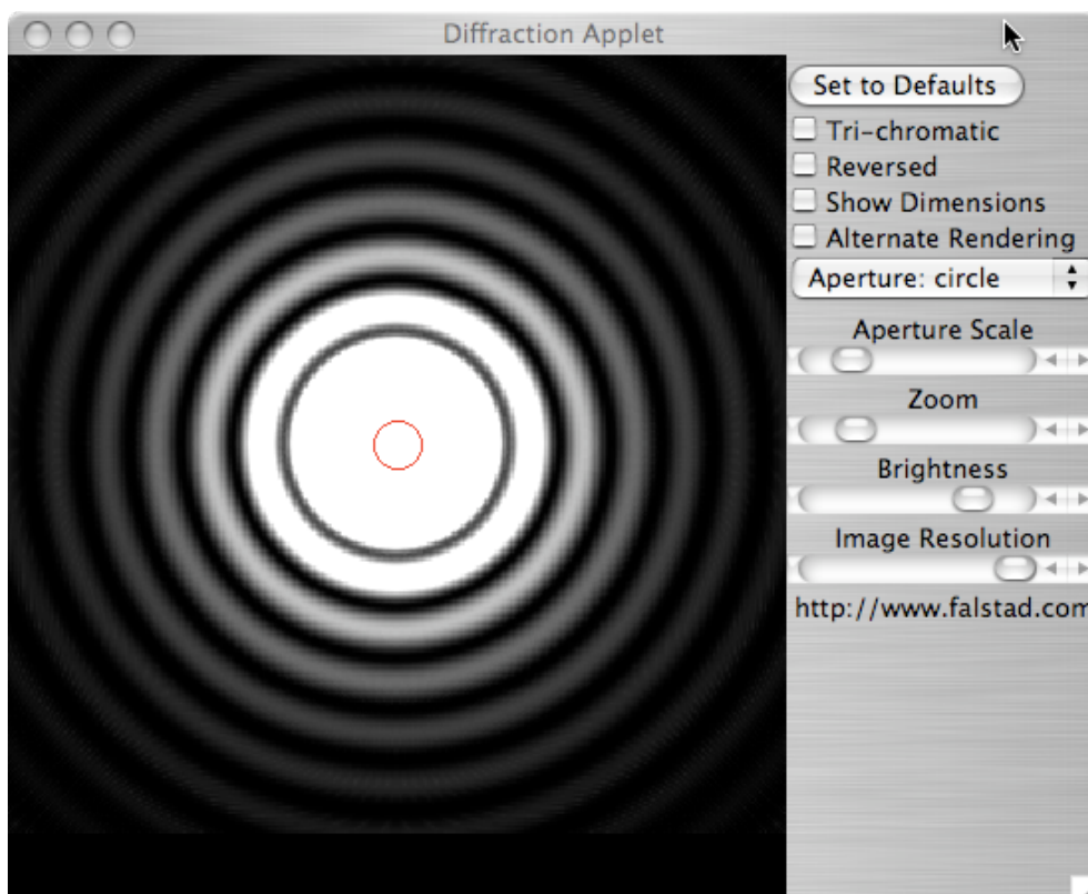
Figure de diffraction obtenue par une ouverture circulaire.
