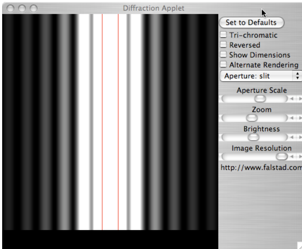
Figure de diffraction obtenue par une fente verticale
